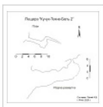
Кучук-Текне-Бель 2 Полуинструментальная съемка
